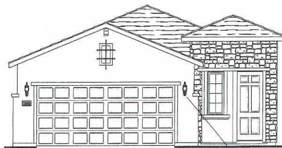
Elevation 'C'
